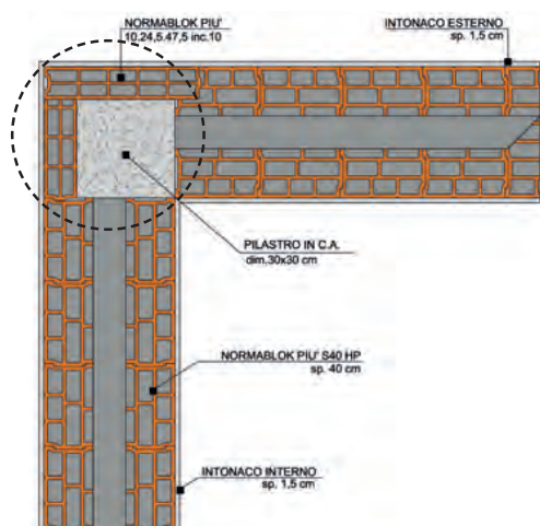
Muratura Normablok Più S40 HP - Pilastro 30x30
