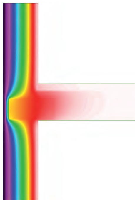
Attacco solaio - Muratura NORMABLOK PIÙ S40 SISMICO
