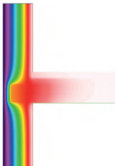
Attacco solaio - Muratura Normablok Più S40 HP
