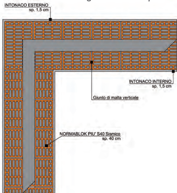
Angolo di muratura portante NORMABLOK PIÙ S40 SISMICO
