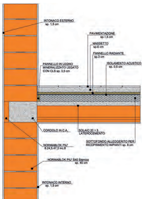
Attacco solaio - Muratura NORMABLOK PIÙ S40 SISMICO
